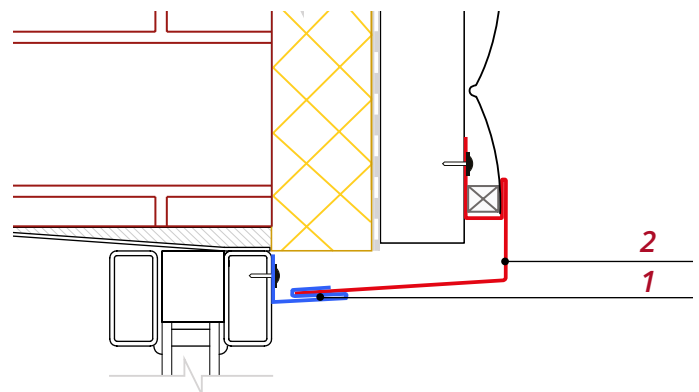
Рис. Верхний откос с Планкой приемной оконной
