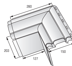
кут відкосу + листва Класик
